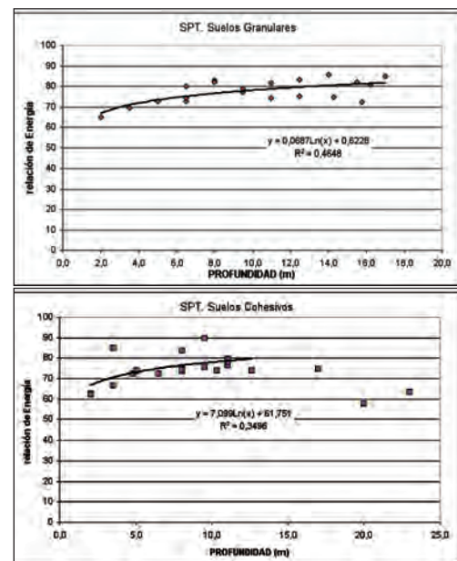
[Fig. 3].- Valores de relación de energía en función de la profundidad para suelos granulares (arriba) y para suelos cohesivos (abajo).
